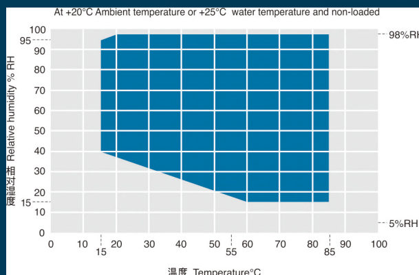
溫濕度控制範圍梯形圖
